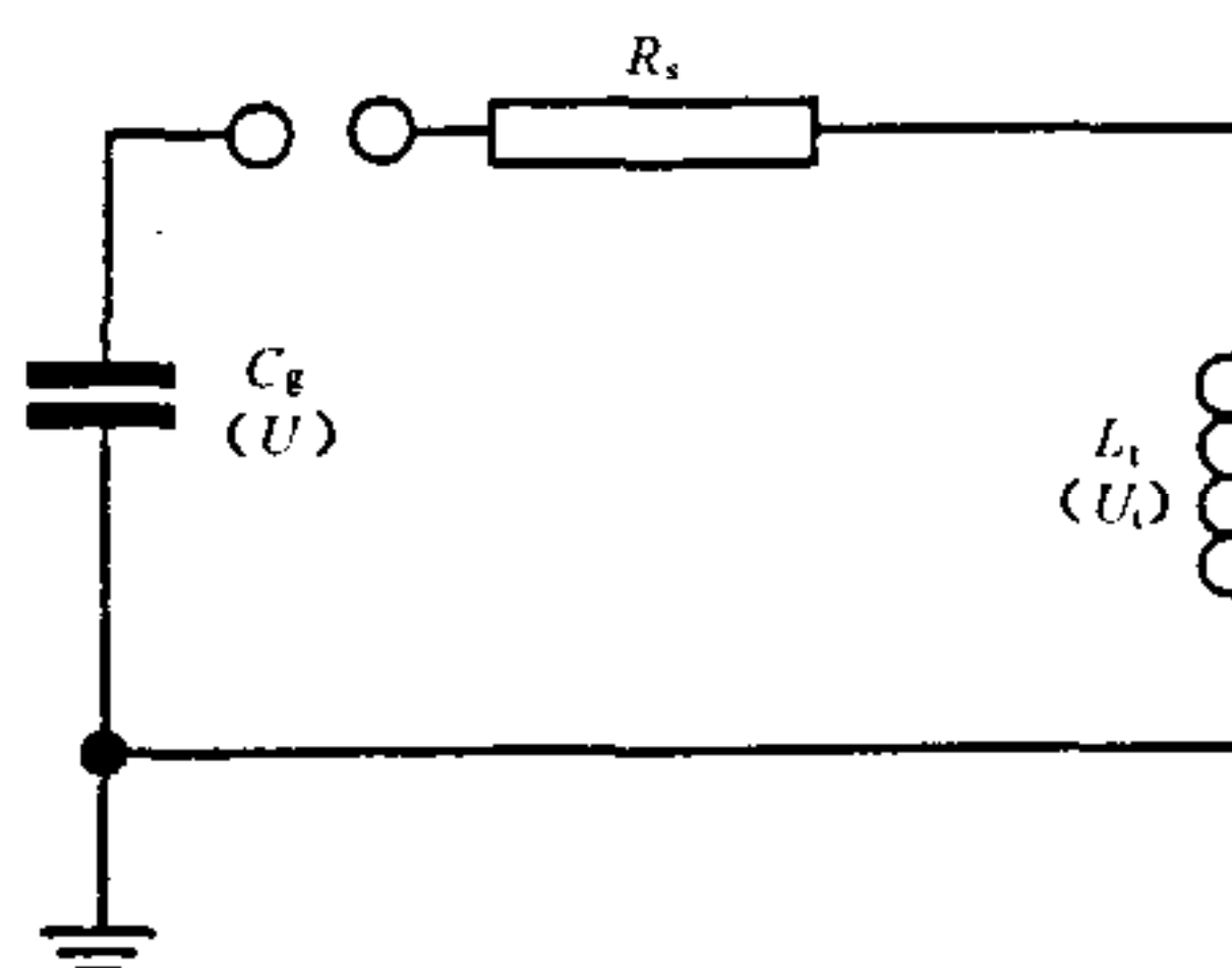
图 A.2 低阻抗绕组的波尾控制
