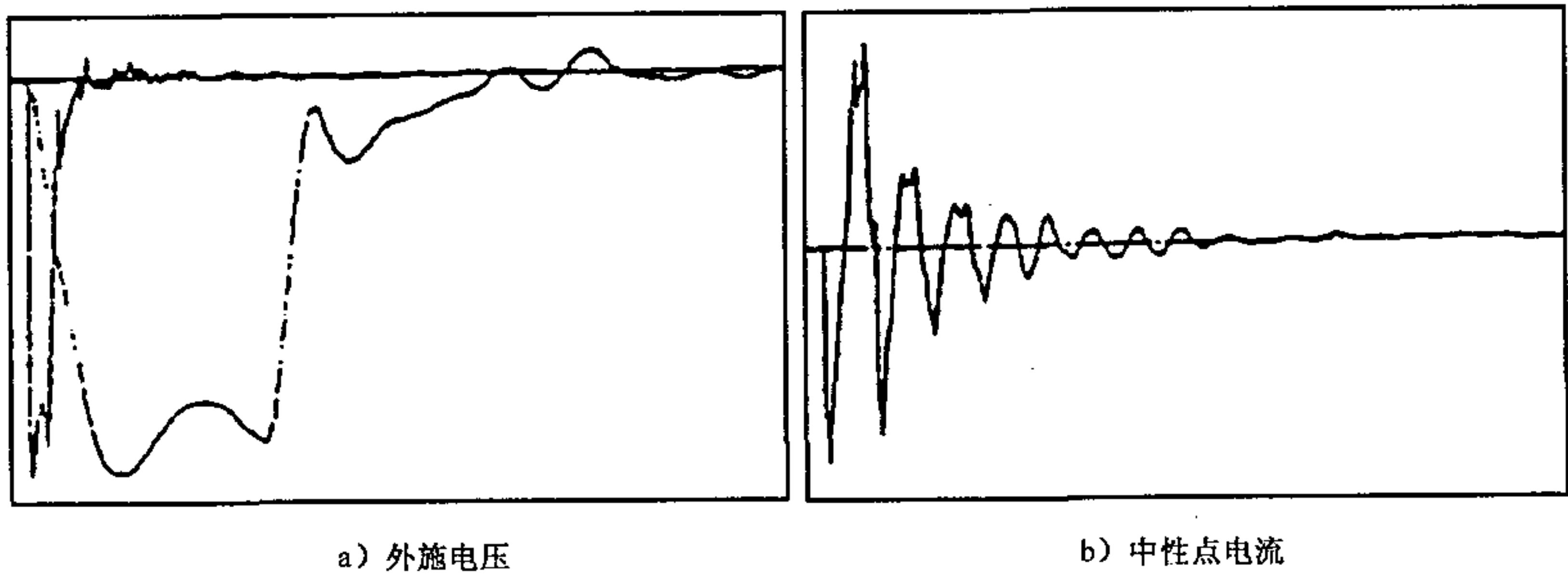
注：层式绕组上的非标准截波。层间阻抗避免了截波对地电压的迅速下降, 也不产生围绕零点的振荡。 图 B. 20 雷电冲击截波——层式绕组的非标准截波
