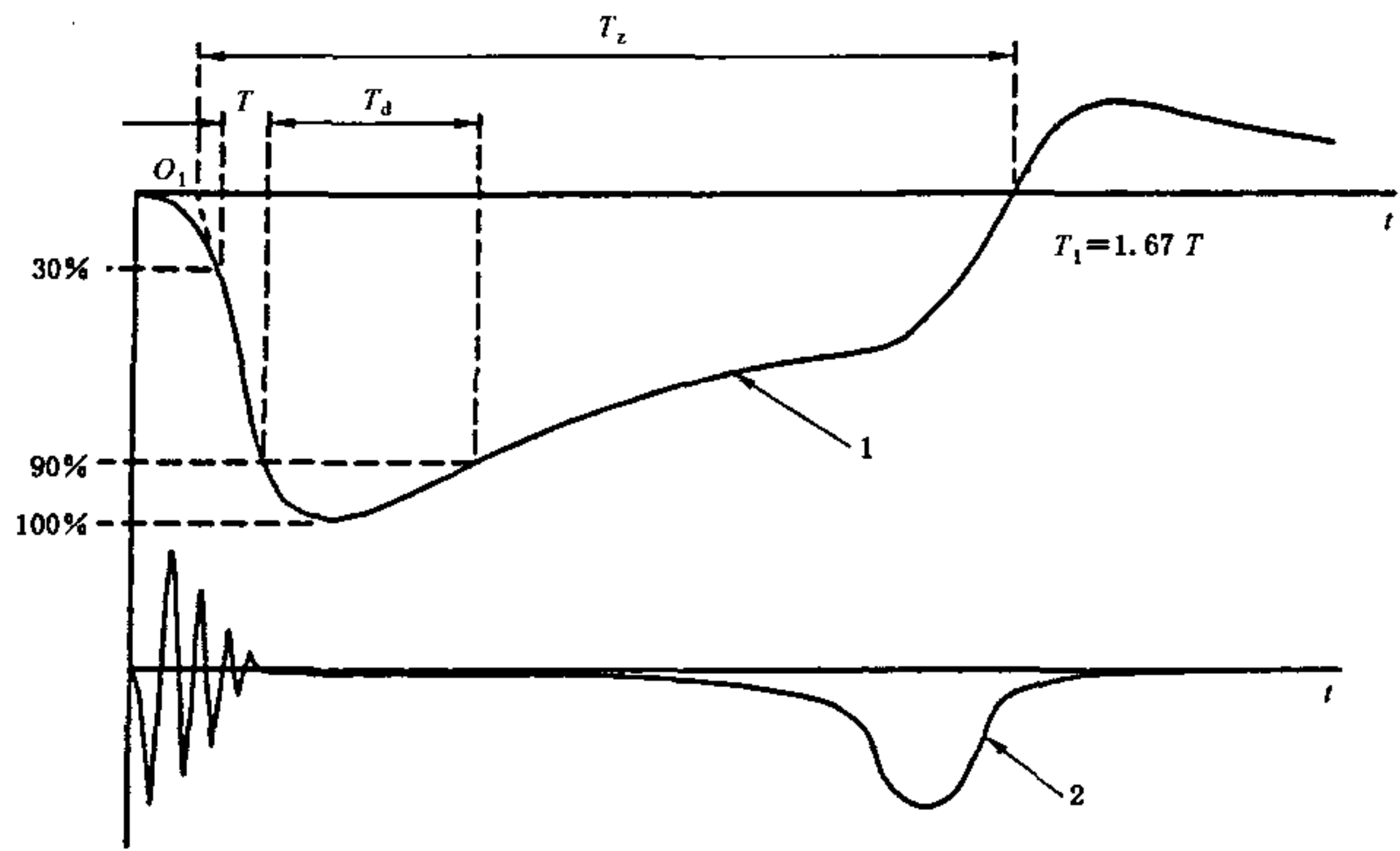
a) 变压器的操作冲击波形 图 3 变压器和电抗器的操作冲击波形
