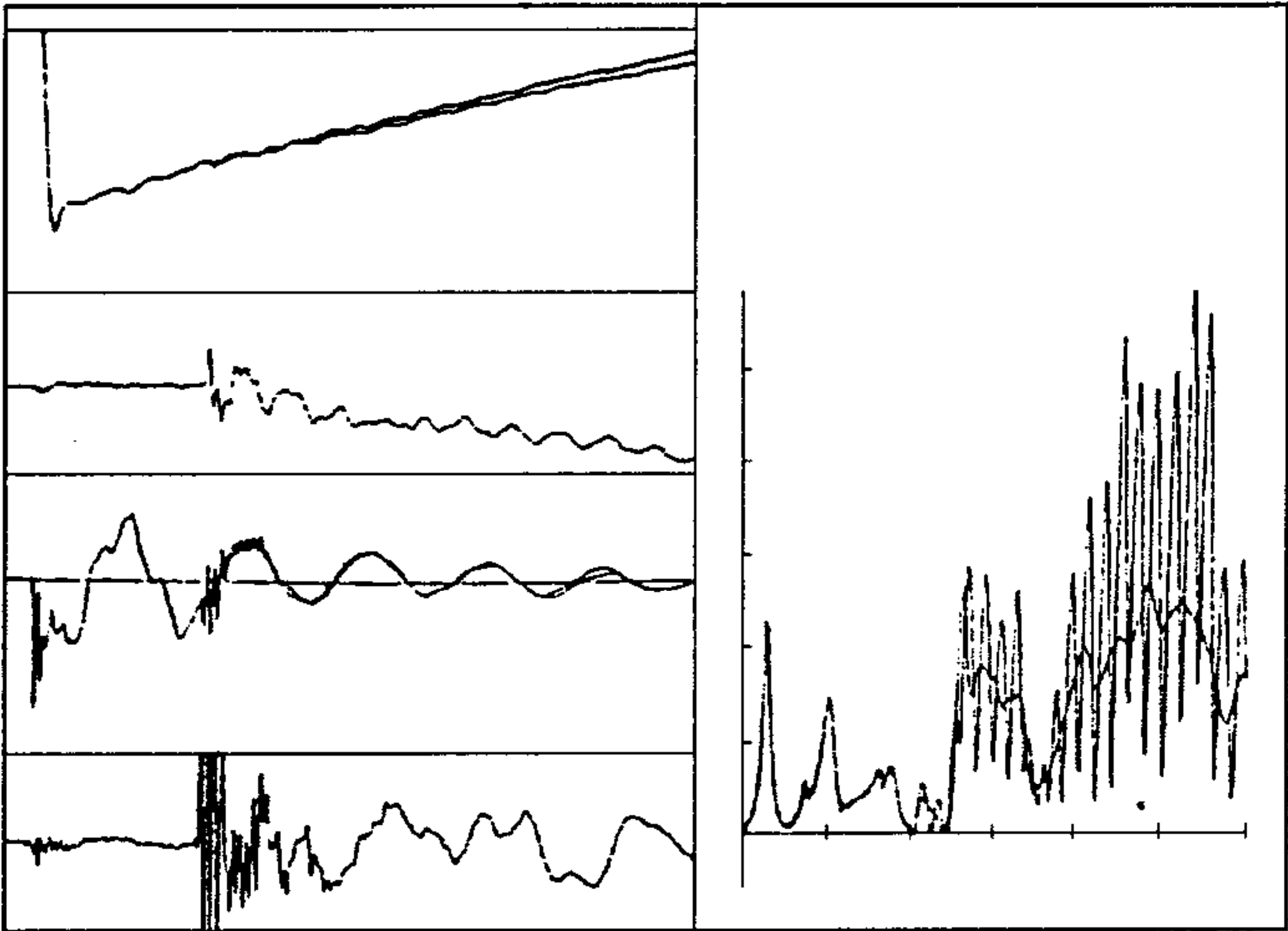
a) 300 MVA, 400/110/30 kV 变压器分接开关引线间的闪络
