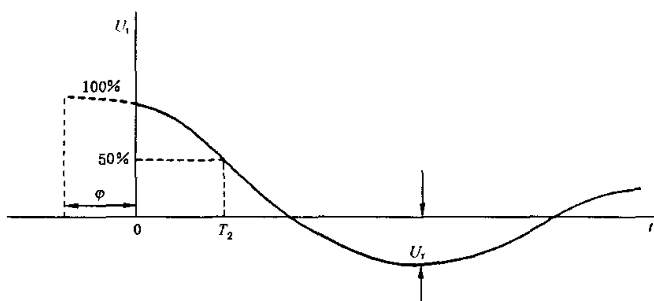
图 A.3 衰减振荡波形图
