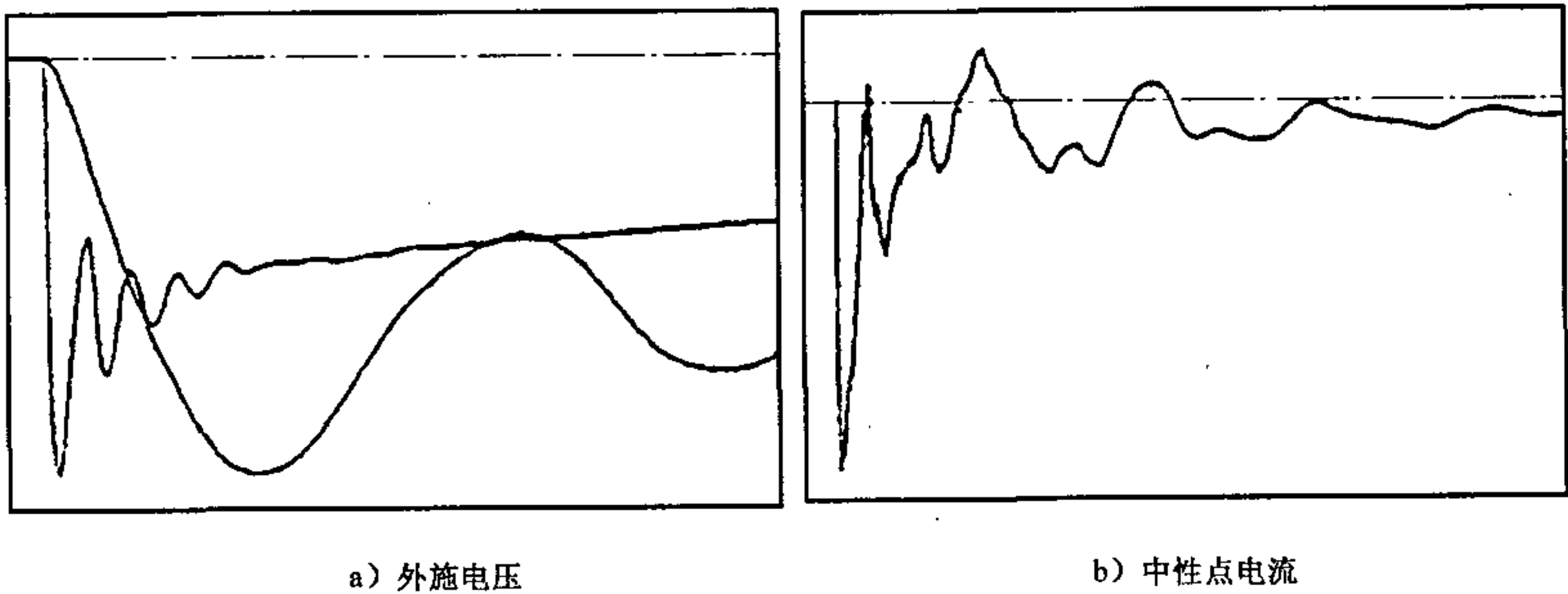
注：根据叠加振荡的第一段波形图, 用数字记录仪估算的半峰值时间为 5 \mu s, 而按 GB/T 16927.1 估算则为 50 \mu s。 图 B. 19 雷电冲击全波——非标准波形, 叠加的振荡波幅值大于 50% 且频率小于 0.5 MHz
