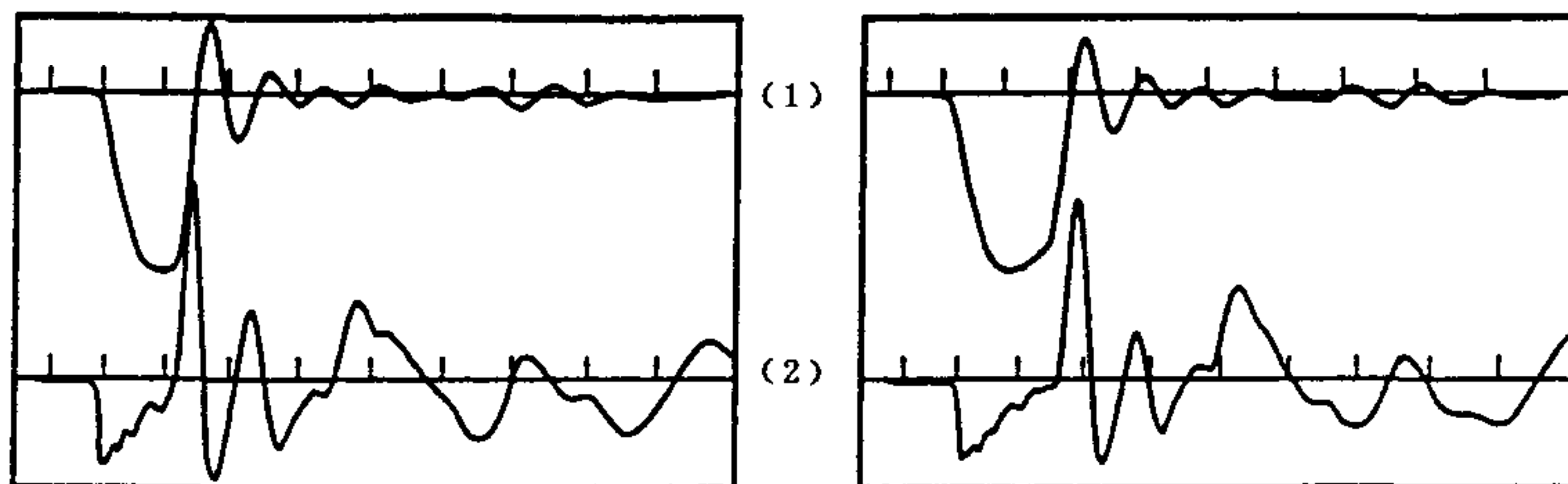
a) 降低电压截波 (62.5%)
