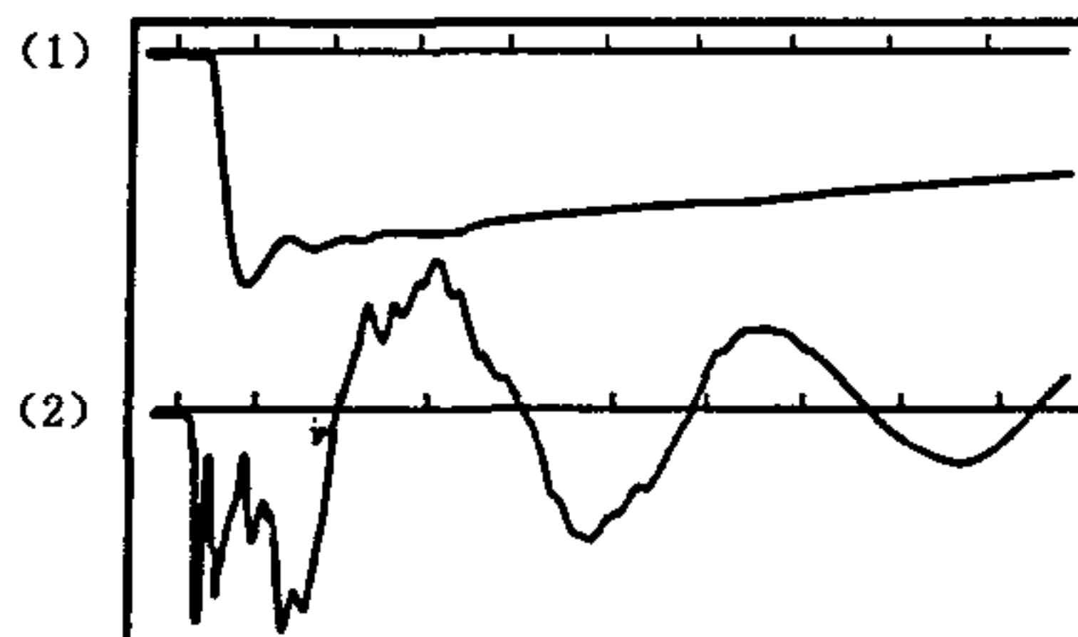
c) 第二个全波 (100%)
