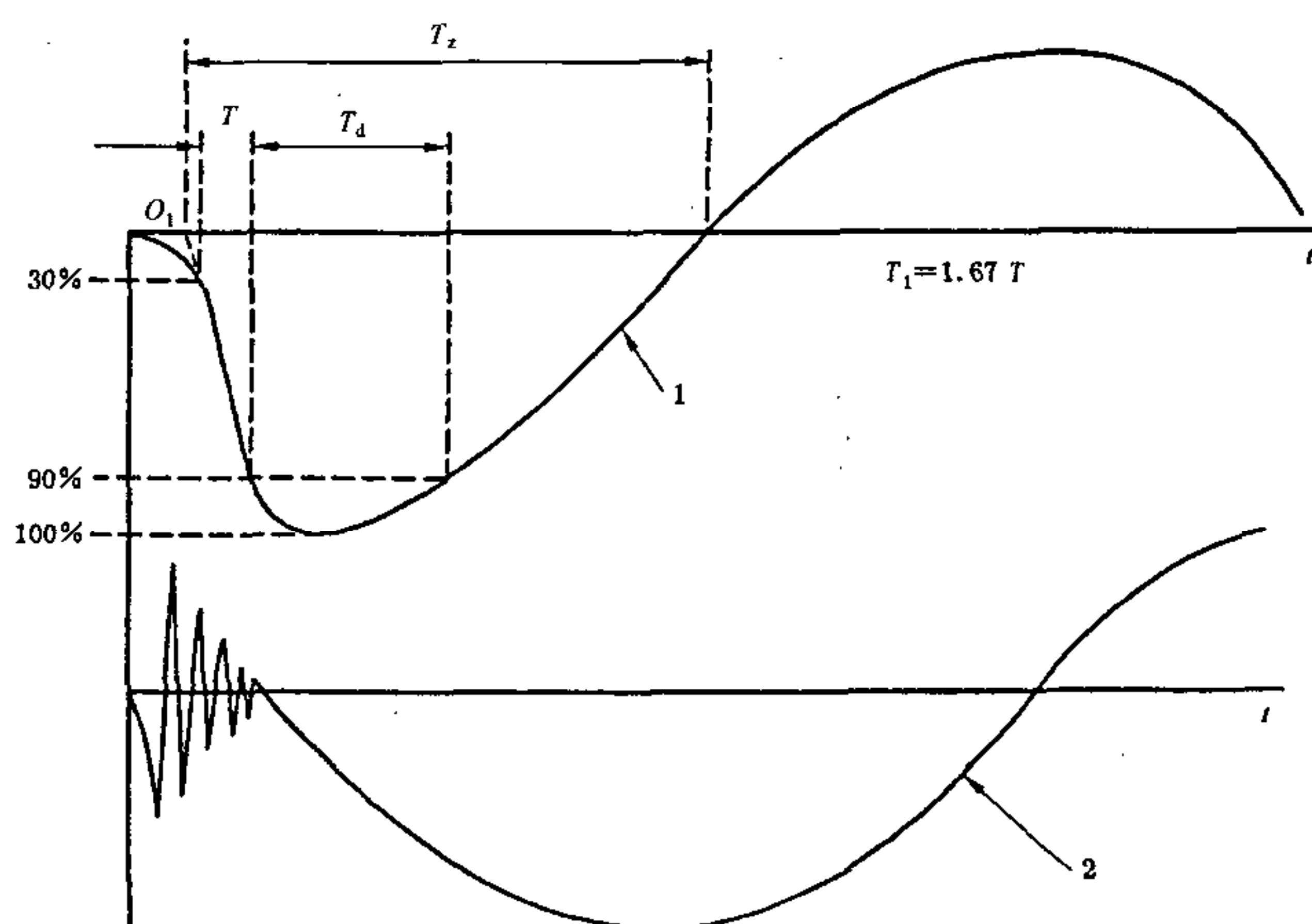
b) 电抗器的操作冲击波形
