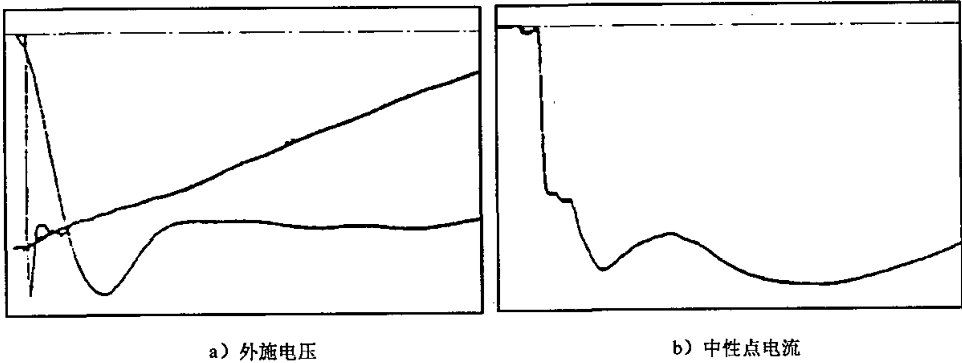
注：按 GB/T 16927.1, 通过波尾下降部分的切线, 估算波形有 19% 的过冲, 故幅值估算误差可能超过 10%。 图 B. 18 雷电冲击全波——非标准波形的估算——数字记录仪中的内置平滑算法的影响
